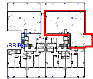
1 Localización local comercial 1 : 1000
